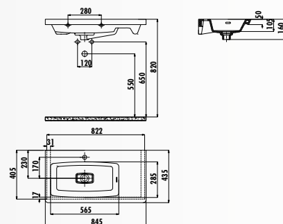
MY085-00CB00E-0000 • Раковина Memory 85 см
